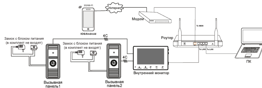
Рис. 1 – проводная схема подключения к сети.
